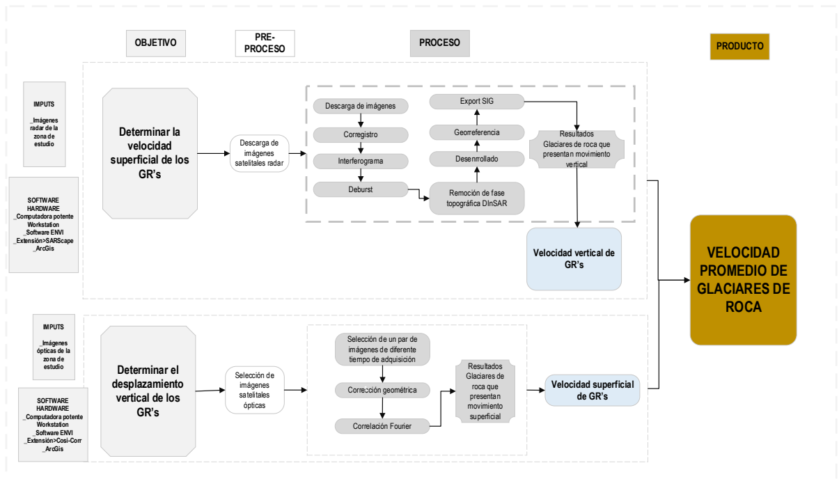
Figura 9. Flujograma de determinación de velocidades superficiales de glaciares rocosos.
