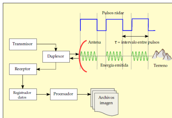
Figura 3. Esquematización del funcionamiento de un sistema RADAR. Fuente, Prieto Morín (2015).
