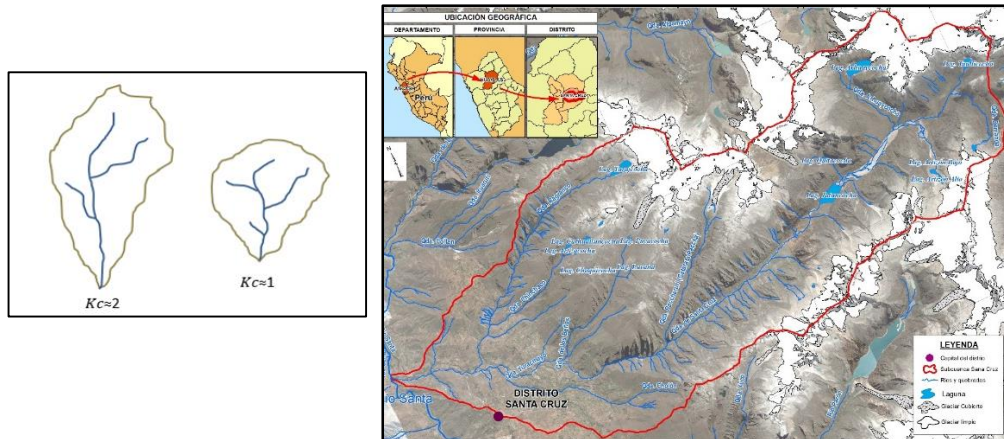
Figura N° 193: (a.) Comparación de la forma de subcuencas según valores del Coeficiente de Compacidad. (b.) Subcuenca del río Colcas con un K_c=1.4560 , caracterizándola como poco alargada.
