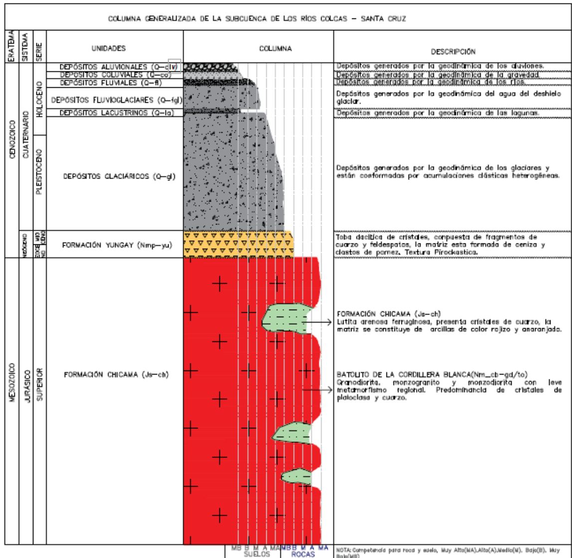
“Año del Diálogo y la Reconciliación Nacional” Figura N° 6: Columna Geológica Generalizada en el Estudio
