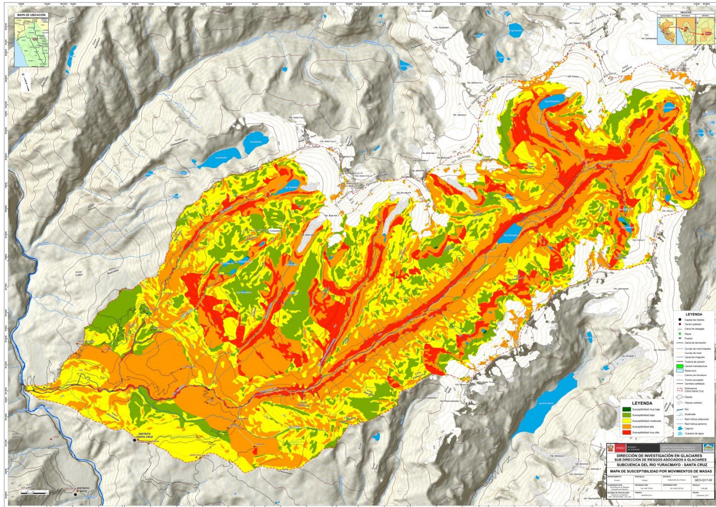
Figura N° 31: Mapa de Susceptibilidades a Movimiento de Masas – Subcuenca del Río Colcas, Quebrada Santa Cruz
